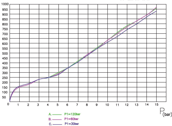
GR-B 流量曲線圖
