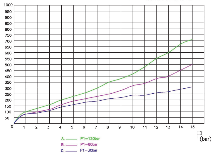
GR-B-V 流量曲線圖
