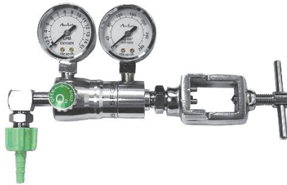
UB-105 (CGA870 結瓶框-雙大錶)
